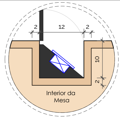
DETALHE RÉGUA DE TOMADAS
