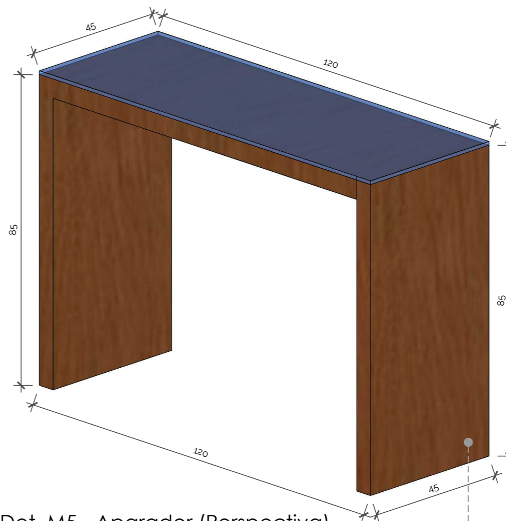
Det. M5 - Aparador (Perspectiva) Esc.: 1/10 5 Unidades
