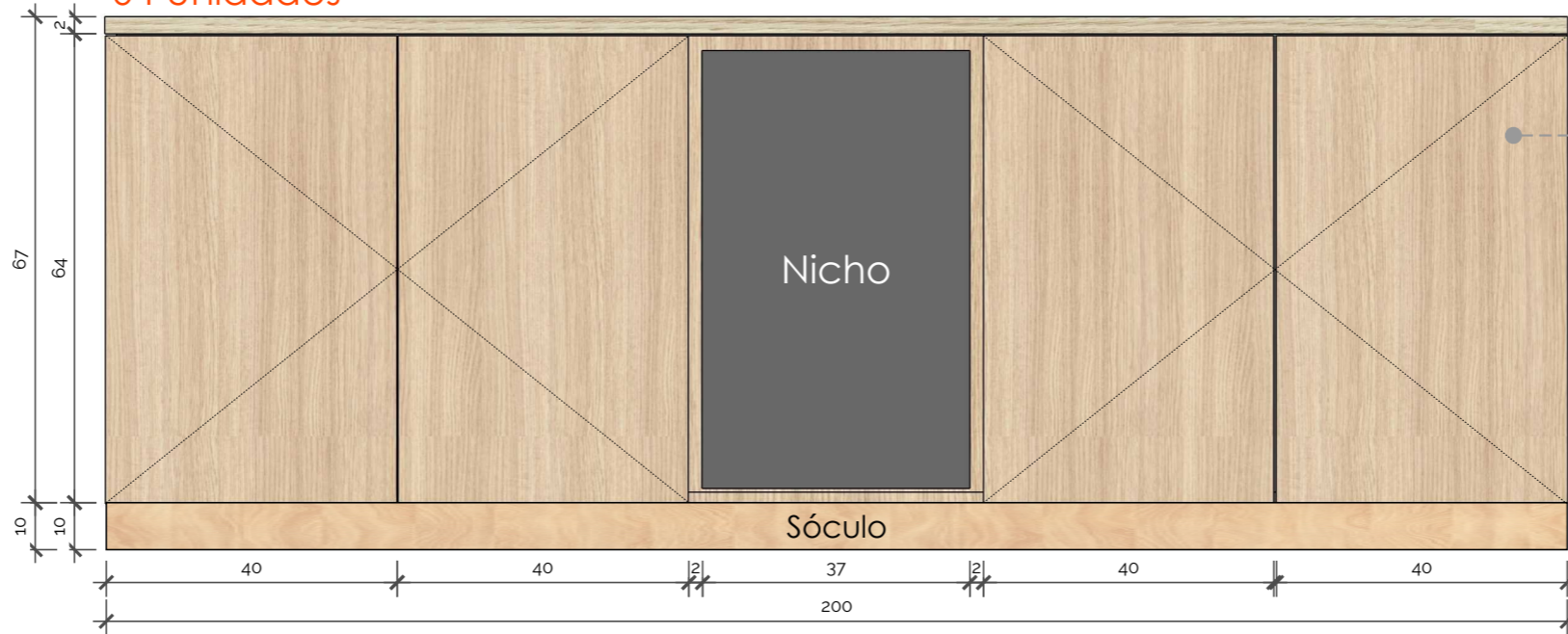
Det. M43 - Armário Baixo (Vista Frontal Externa)
