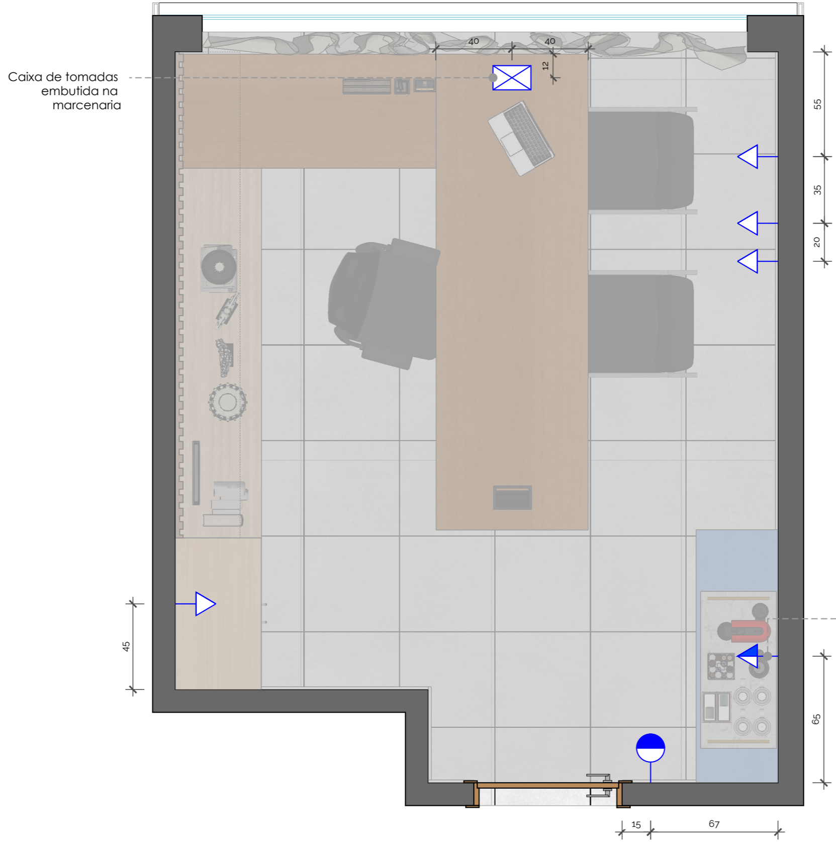
Planta de Pontos Sala da Presidência Esc.: 1/20
