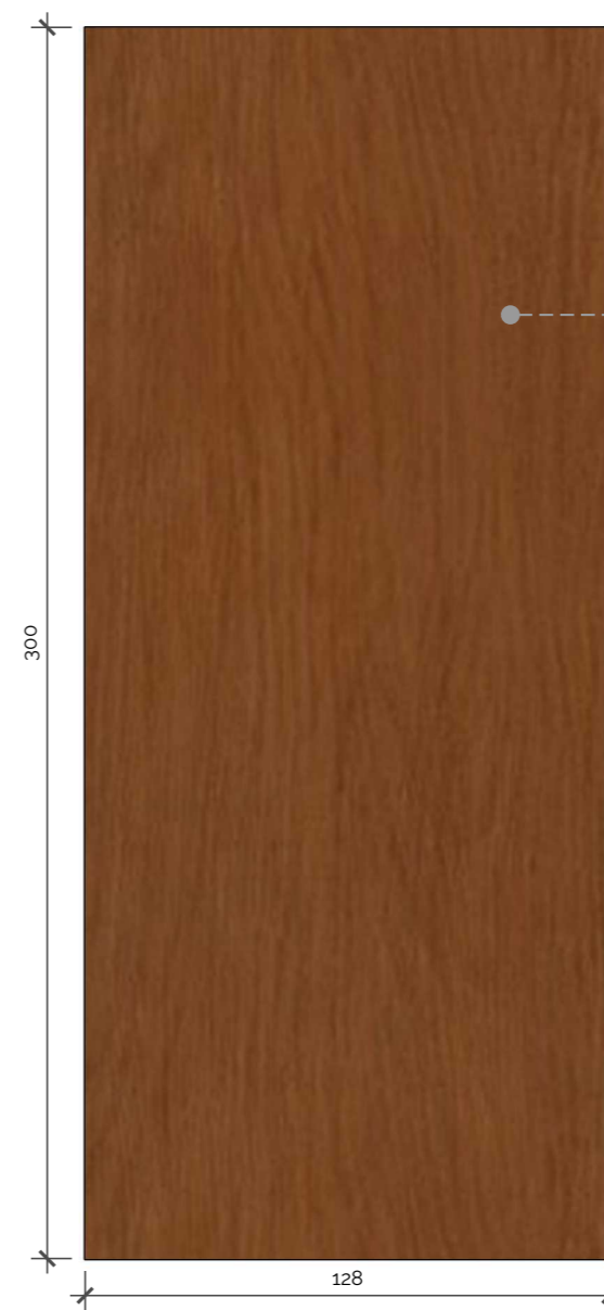
Det. M38 - Painel em "U" (Vista C) Esc.: 1/20 01 Unidade
