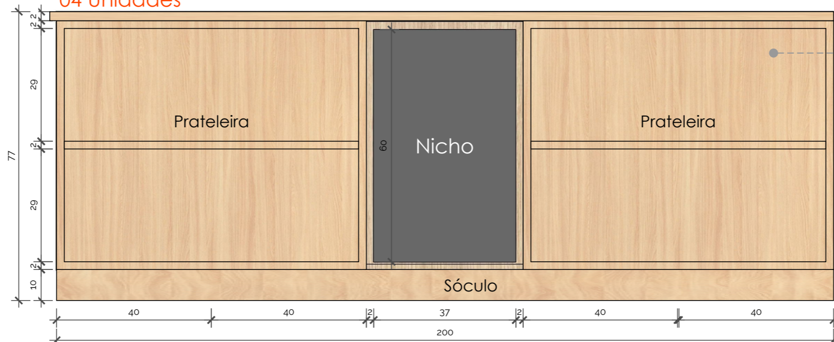
Det. M43 - Armário Baixo (Vista Frontal Interna)
