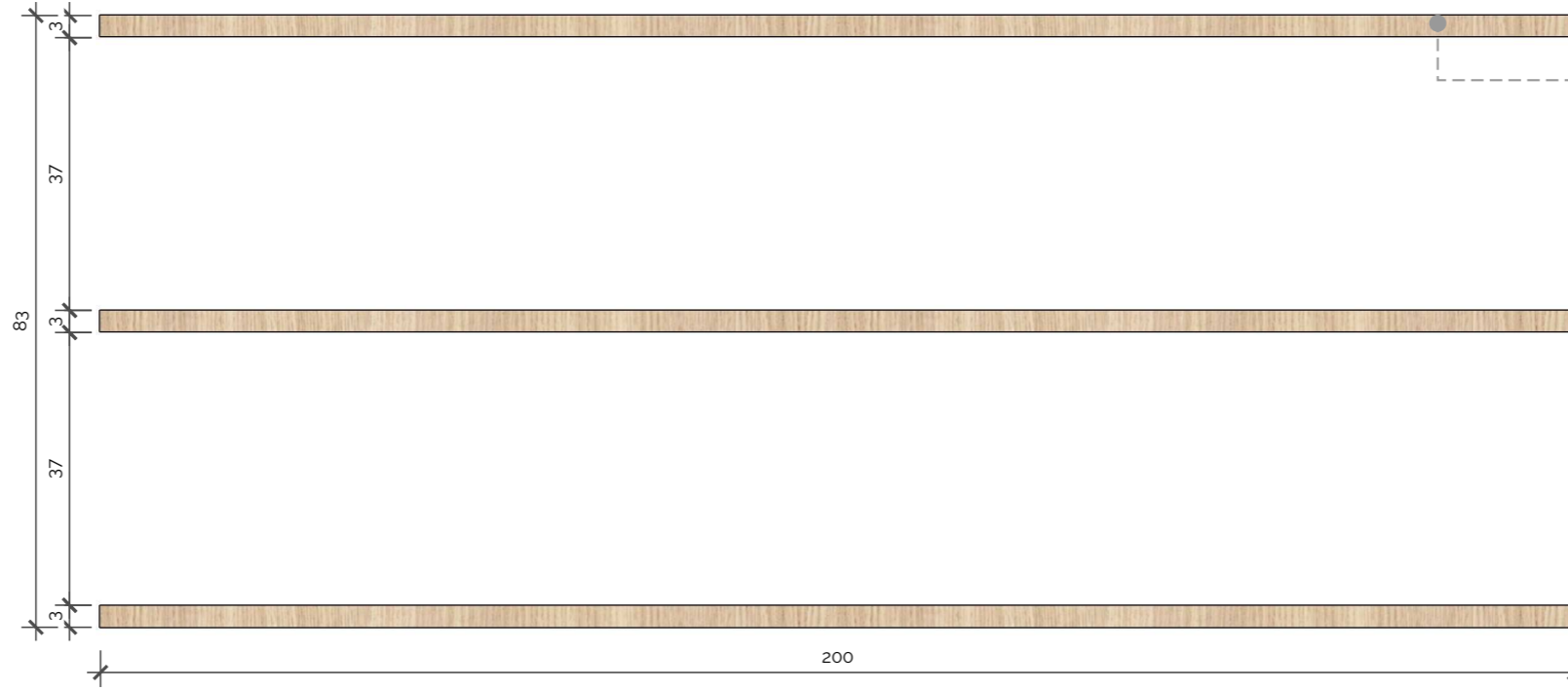
Det. M45 - Painel (Vista Frontal) Esc.: 1/10 04 Unidades
