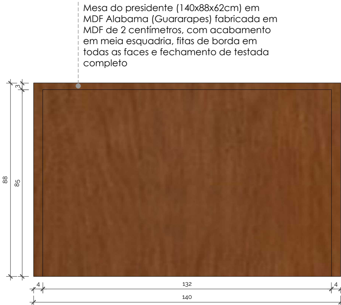
Det. M7 - Mesa de Presidente (Vista Frontal) Esc.: 1/10 01 Unidade
