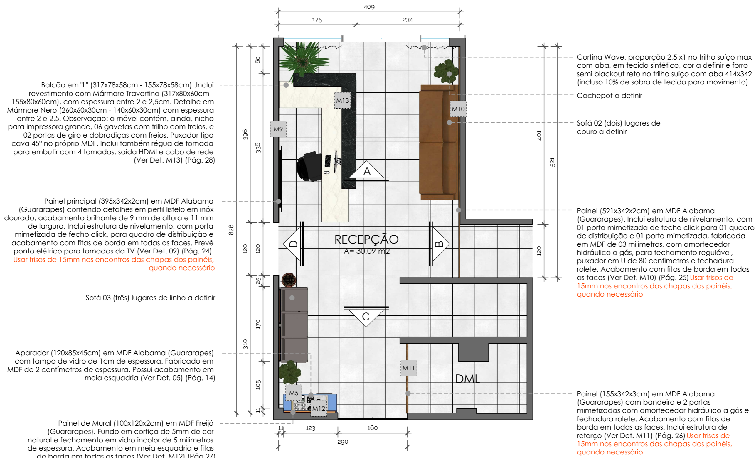
Planta Layout Recepção Principal Esc.: 1/50
