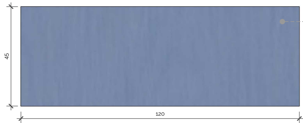
Det. M5 - Aparador (Vista Superior) Esc.: 1/10 5 Unidades
