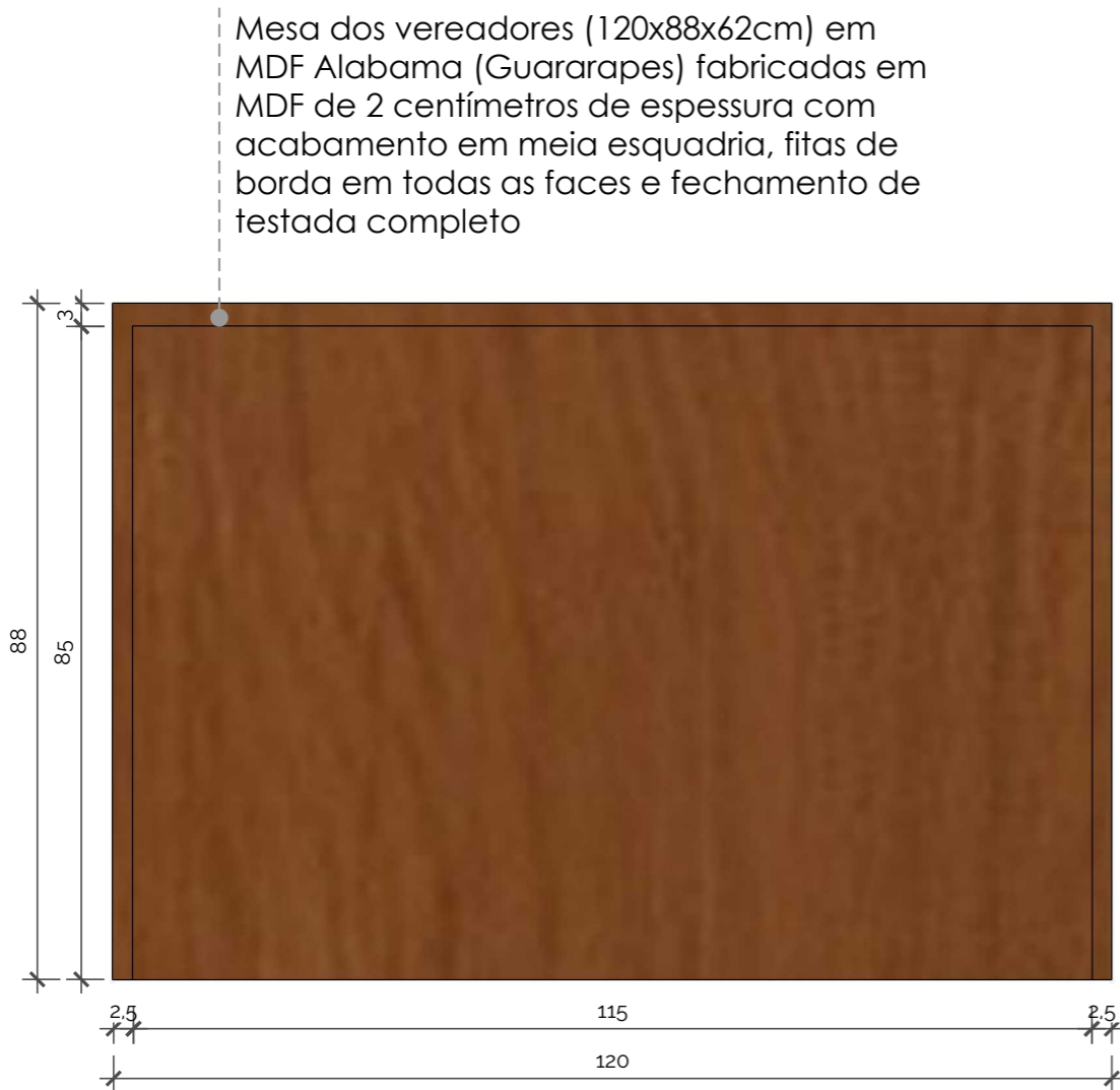
Det. M6 - Mesa de Vereadores (Vista Frontal) Esc.: 1/10 10 Unidades
