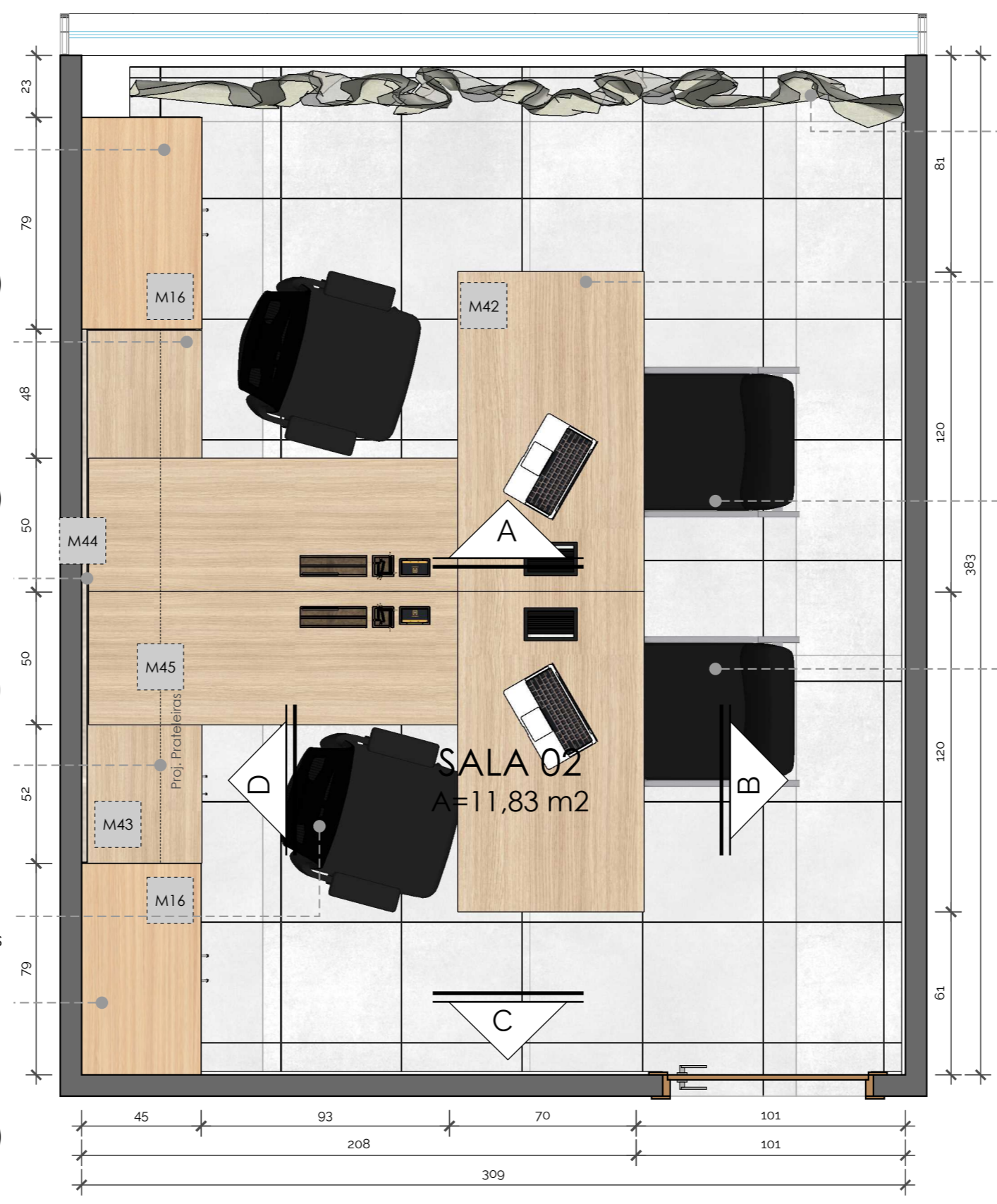
Planta Layout Sala 02 Esc.: 1/20
