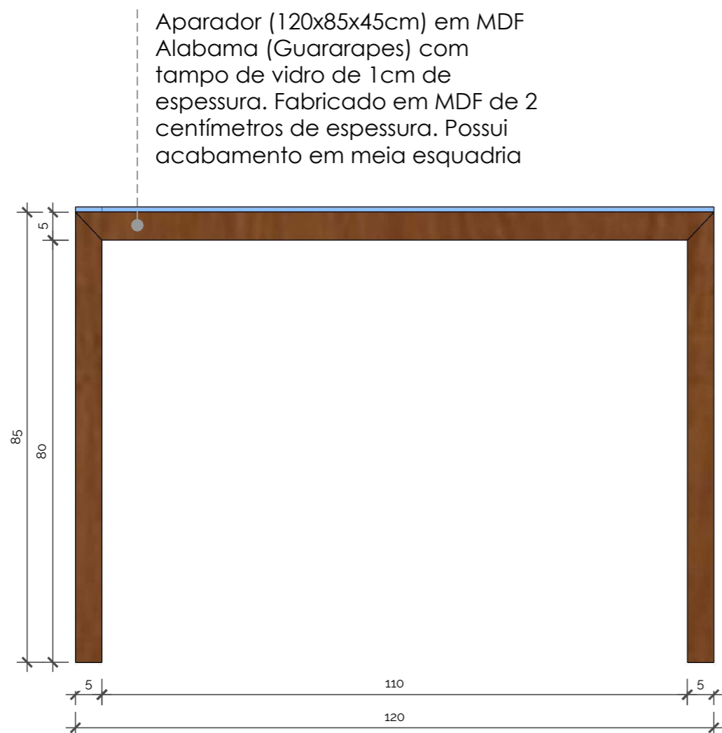
Det. M5 - Aparador (Vista Frontal) Esc.: 1/10 5 Unidades
