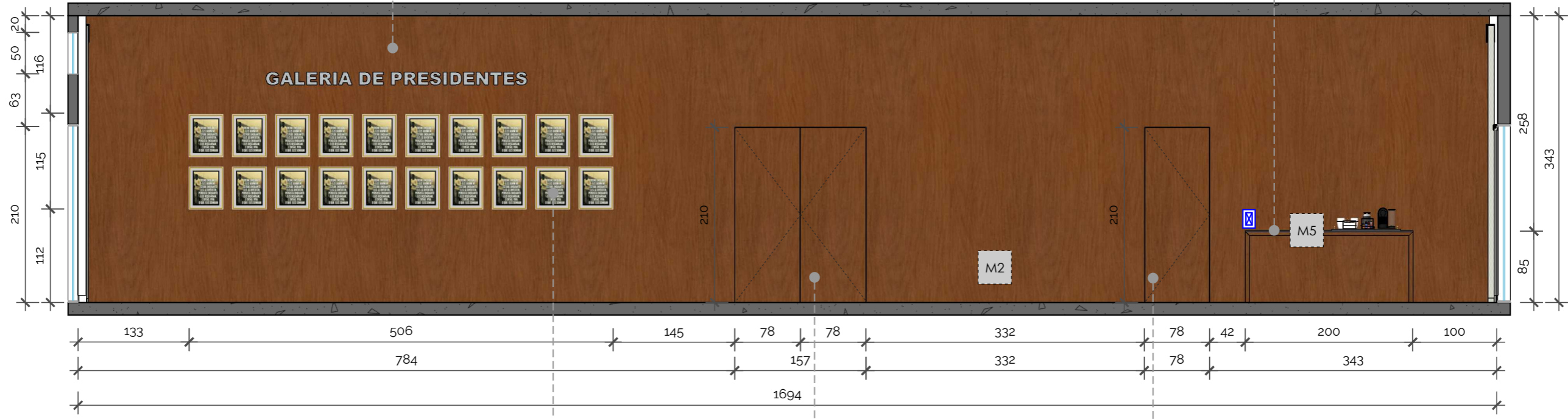
Vista A - Plenário Esc.: 1/55
