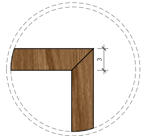
DETALHE MEIA ESQUADRIA
